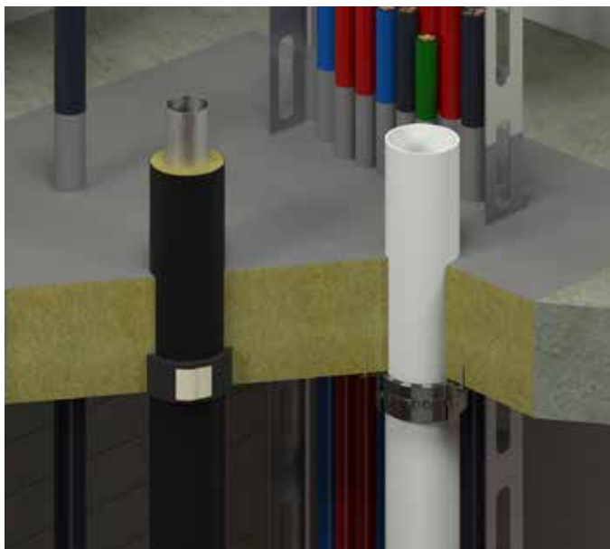
Système PROMASTOP®-CC
